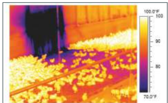
Los ventiladores, inlets o ventanas no tienen la misma capacidad aislante que las paredes. Estas estructuras pueden crear áreas que no son confortables para las aves. Cortesía de M. Czarick – UGA
