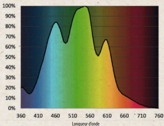
Spectre de la vision lumineuse des oiseaux
