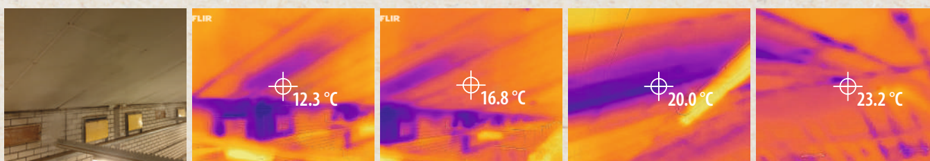
Un bon système de ventilation transversale a pour but de réchauffer l'air entrant en le dirigeant vers le toit où la température de l'air est plus élevée. Cette séquence d'images thermiques nous montre l'effet d'une ventilation transversale optimale.
