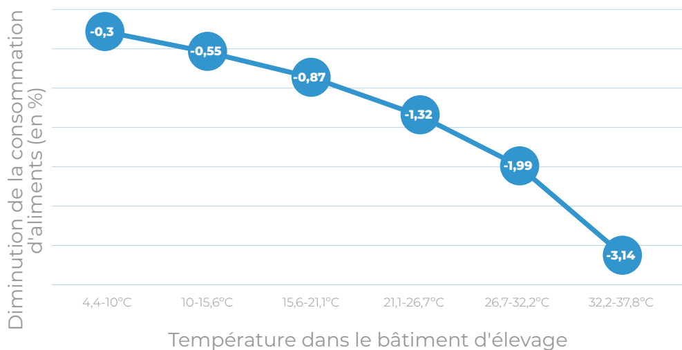
Figure 4. Diminution de la consommation journalière (en %) due à la variation de la température moyenne (1°C) à l'intérieur du bâtiment
