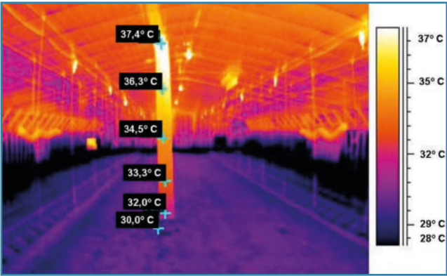
Temperatura siempre tiene una gradiente vertical lo que es un aspecto crítico en sistemas de jaulas. Cortesía de M. Czarick – UGA
