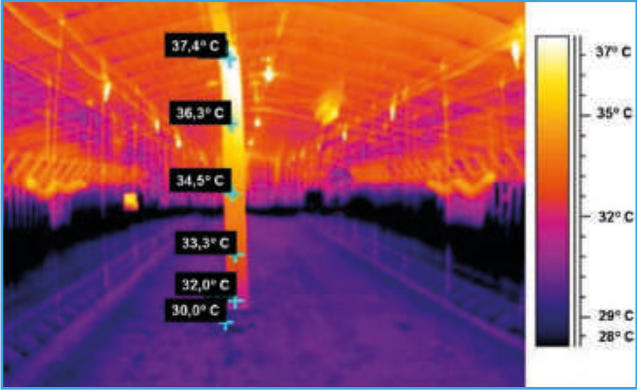
Temperatura siempre tiene una gradiente vertical lo que es un aspecto critico en sistemas de jaulas. Cortesía de M. Czarick – UGA
