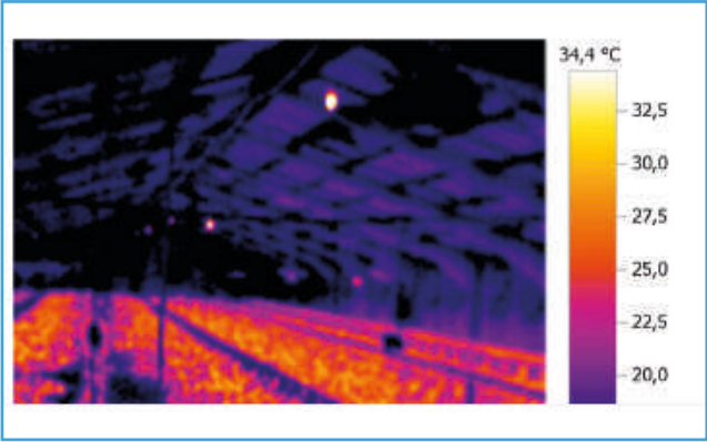
El aislamiento del techo es clave para una correcta temperatura y ventilación de la nave, tanto para climas fríos como cálidos. Cortesía de M. Czarick – UGA
